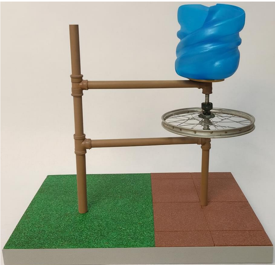
Figura 1. Representação 3D do protótipo.
