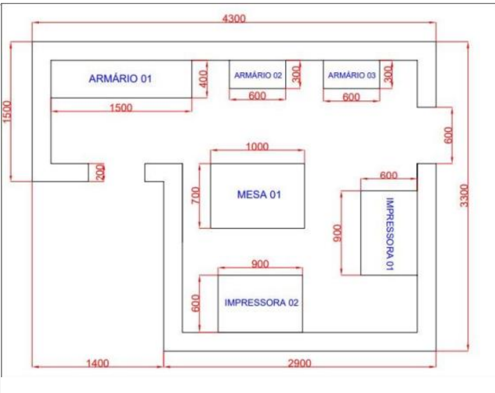
Figura 2. Layout atualizado
