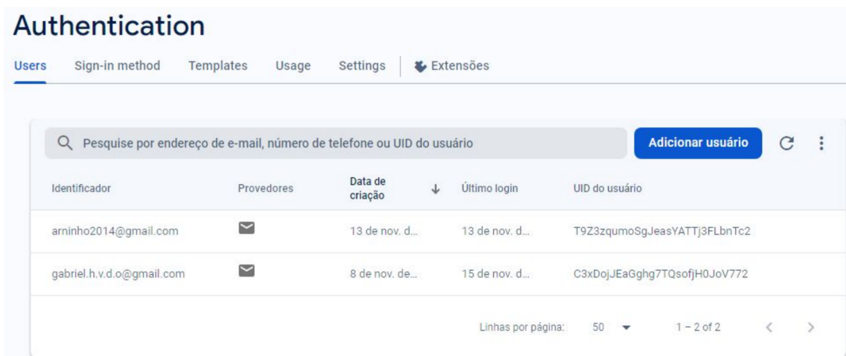
Figura 3. Autenticação Firebase
