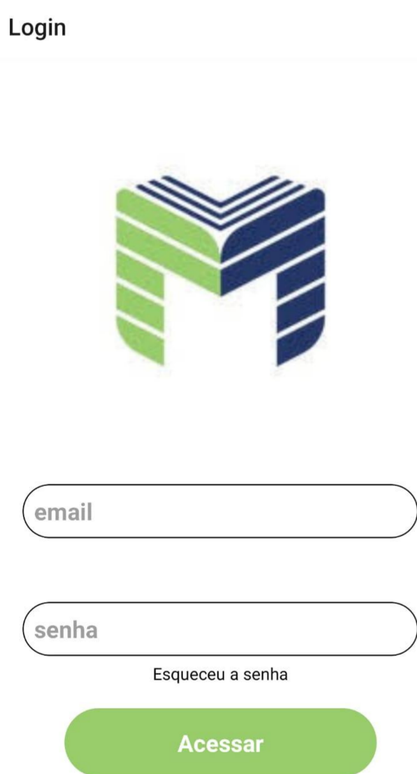
Figura 1. Tela login
