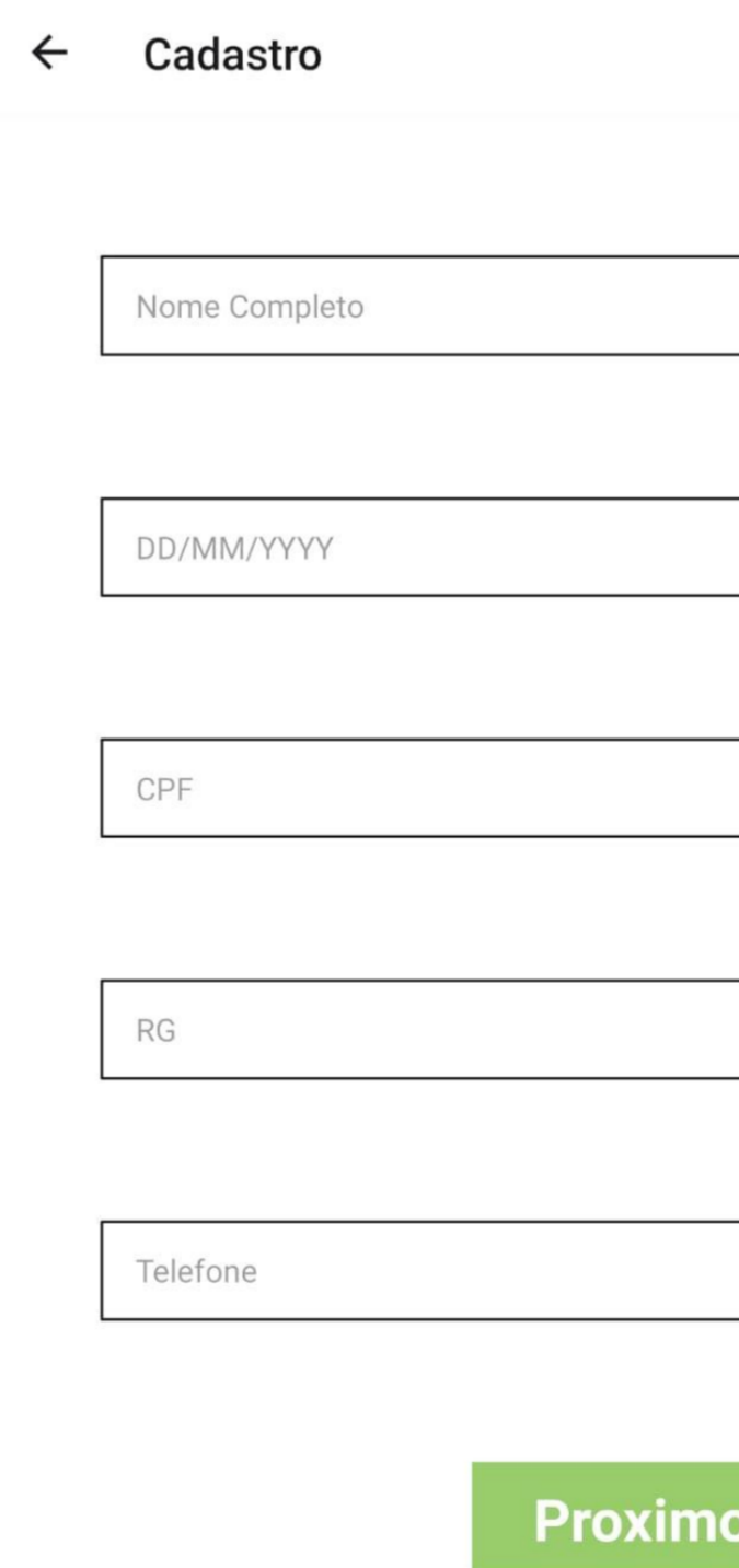
Figura 4. Efetuar Cadastro
