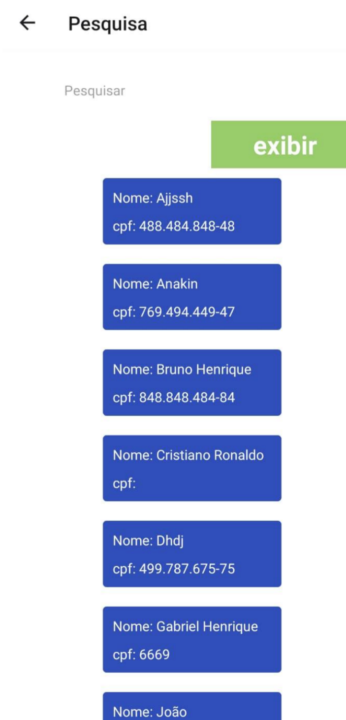
Figura 5. Cadastros
